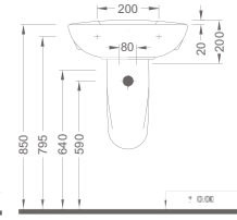
REVNA Yarım Ayak | Half Pedestal
